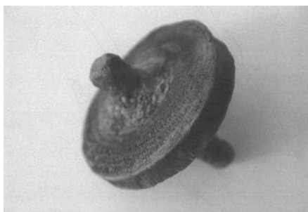
Houten wiel, eiken met geleidingsgroef, rond 75 mm, asje van ijzer, lang 80 mm, lange zijde rond 13 mm, korte zijde vierkant 12 mm.
